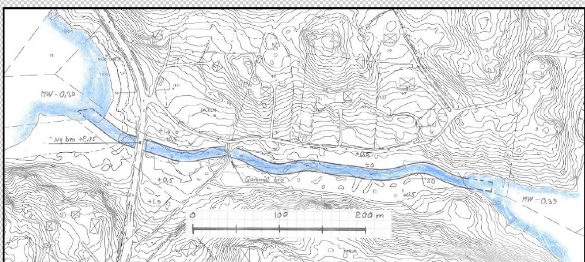
Figur 5 Kanalsträckning
